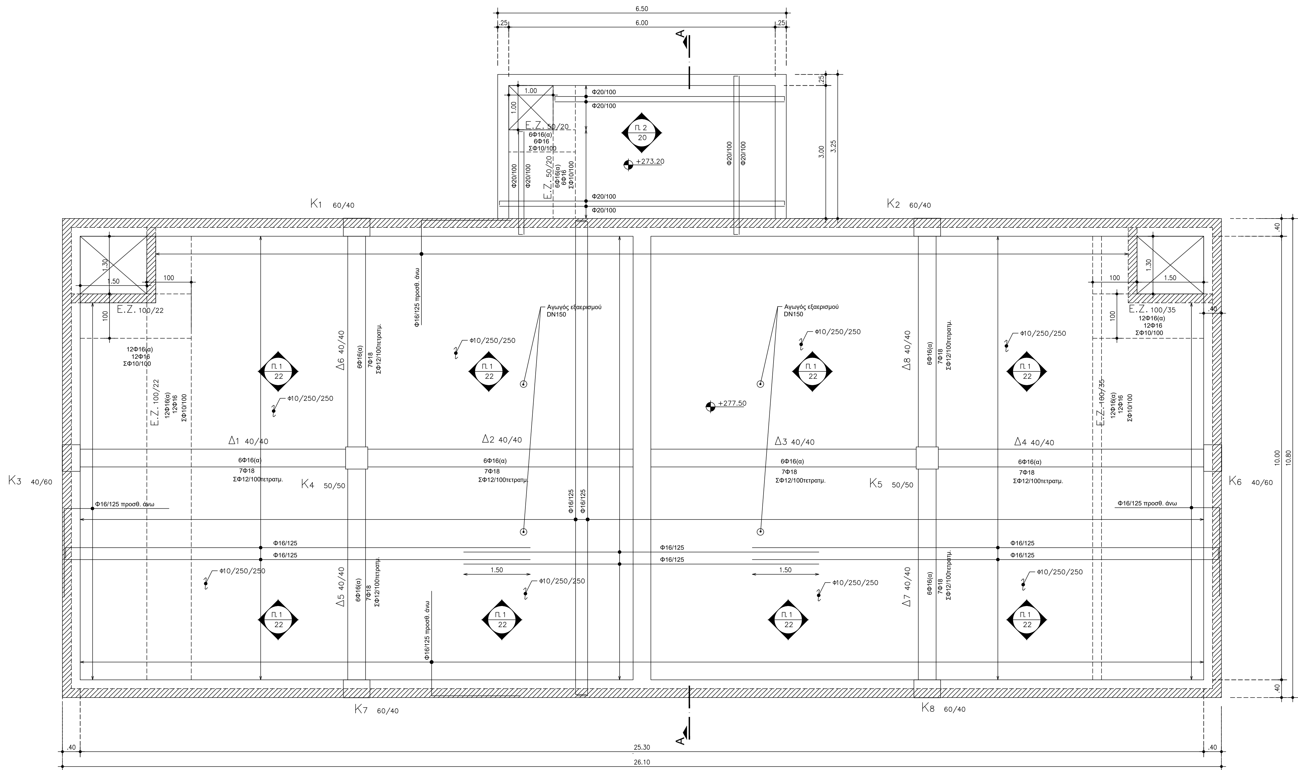
ΟΠΛΙΣΜΟΙ ΔΩΜΑΤΟΣ ΚΛ. 1:50
