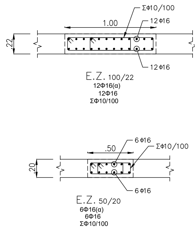
ΛΕΠΤΟΜΕΡΕΙΕΣ ΕΝΙΣΧΥΜΕΝΩΝ ΖΩΝΩΝ ΚΛ. 1:25
