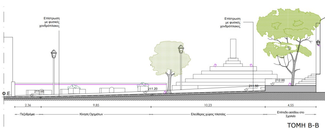
Εικόνα 7. Τομή Β-Β, Η πλατεία και ο δρόμος κίνησης οχημάτων
