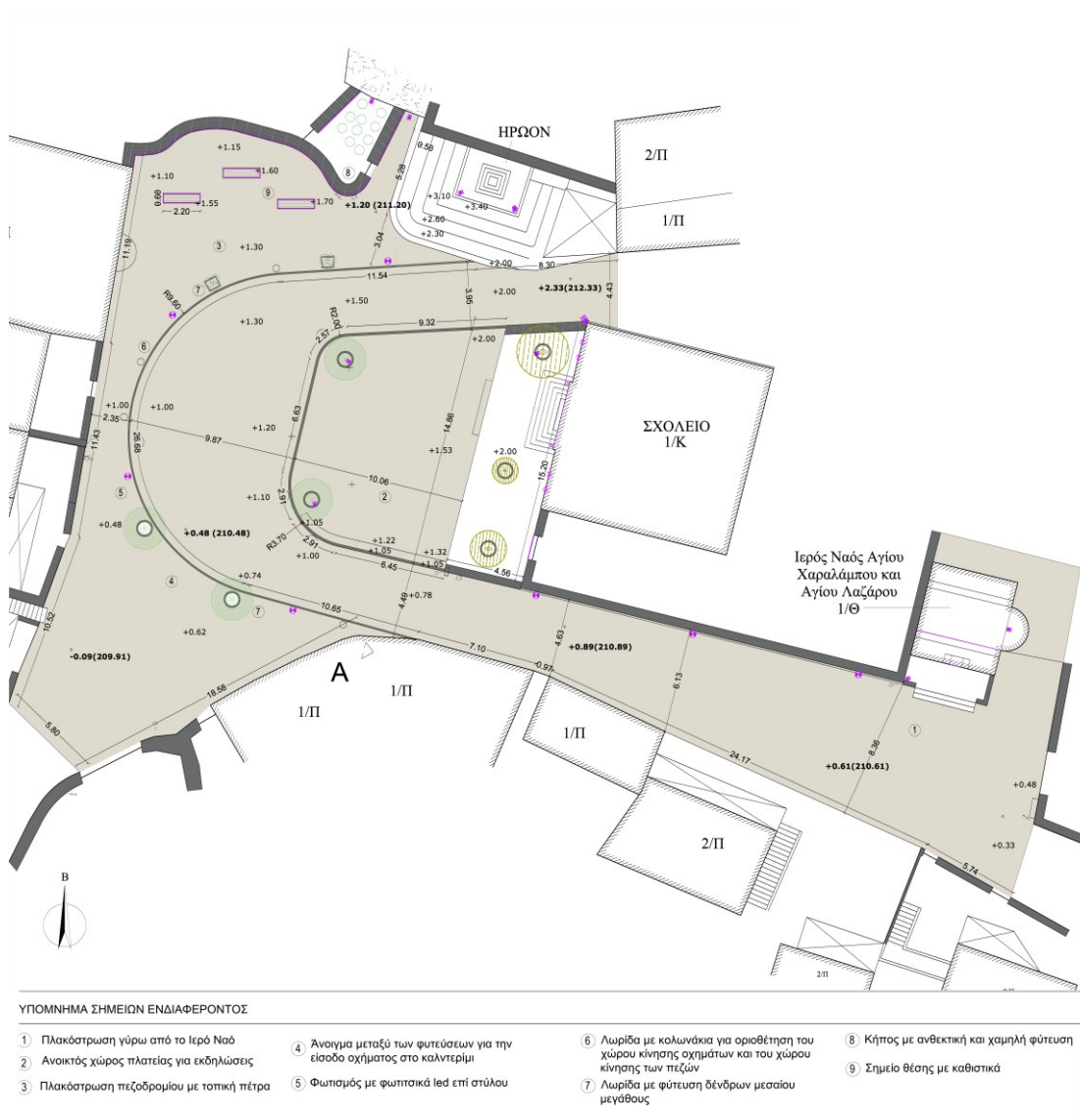
Εικόνα 4. Κάτοψη περιοχής μελέτης
